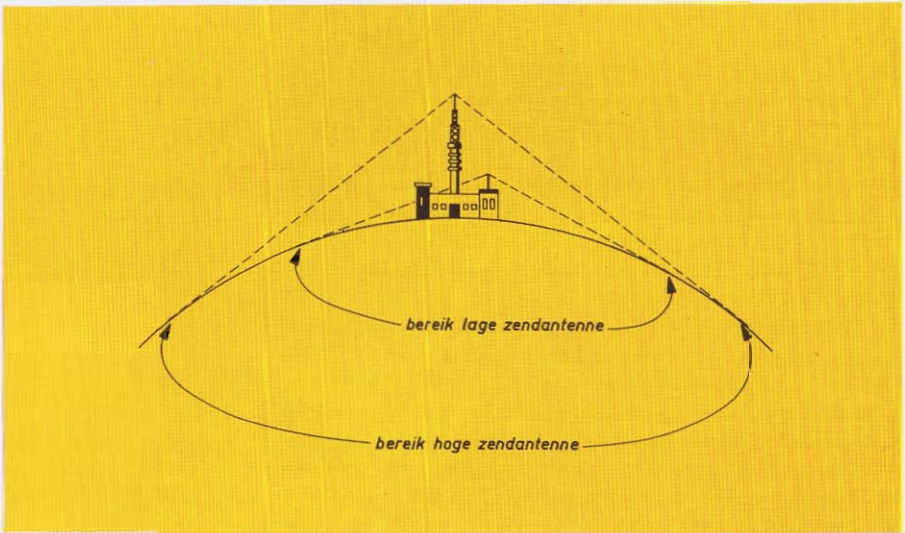
Fig. 8. Zenderbereik voor ultrakorte golven
