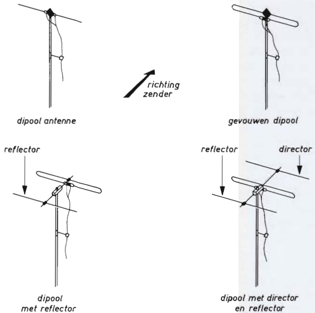
Fig. 10. Verschillende uitvoeringen van FM-kortegolfantennes
